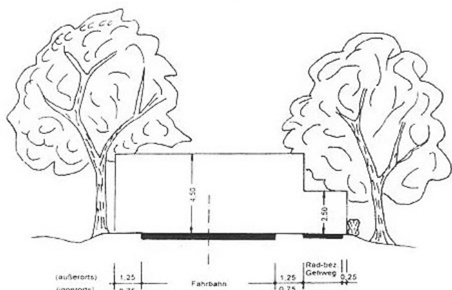
Lichtraumprofil
